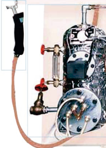
Pistola smacchiatrice aria - vapore Steam-air spotting gun Pistolet de détachage air-vapeur Dampf-Luft-Detachierpistole Pistola quitamanchas aire-vapor
