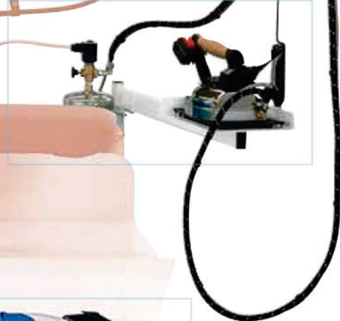
Gruppo ferro vapore completo Complete steam iron assembly Groupe fer vapeur complet Komplette Dampfbügeleiseneinheit Grupo plancha vapor completo
